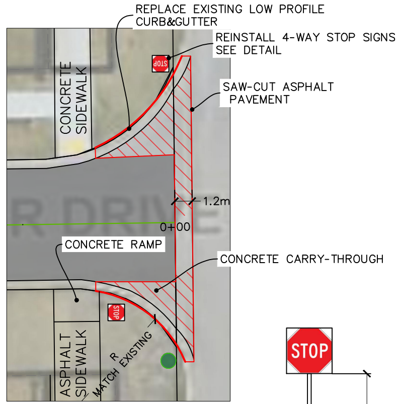
DETAIL A SCALE: 1:250
