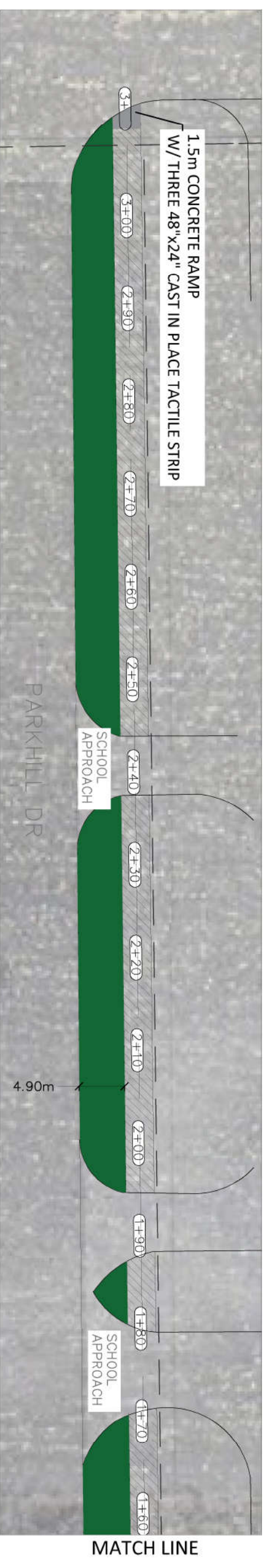
PARKHILL DR SIDEWALK STA 1+60 TO 3+12 SCALE: NTS
